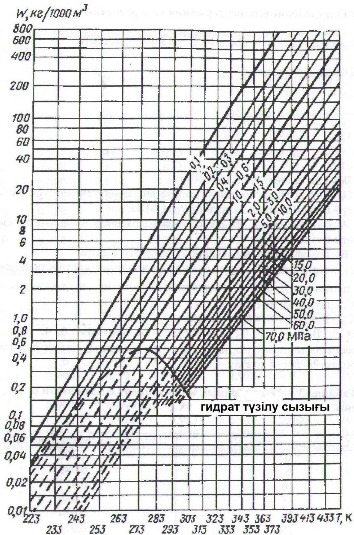
2-сурет. Тұщы сумен өзара әсерлесуі бар газ құрамындағы су буының тепе-теңдік мөлшерінің номограммасы.
